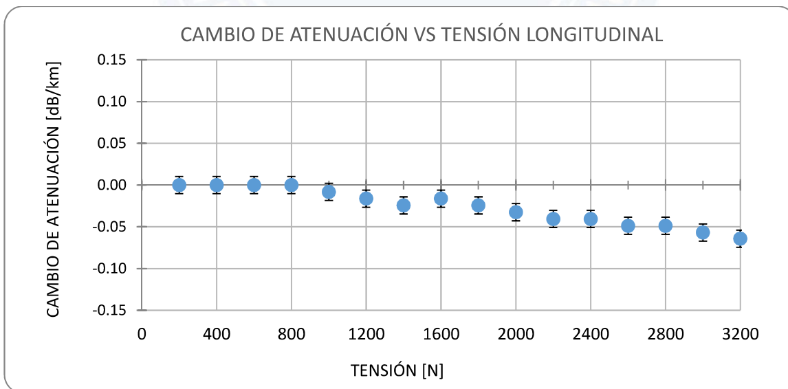
Figura 3. Cambio de atenuación del cable bajo ensayo en función de la tensión aplicada
