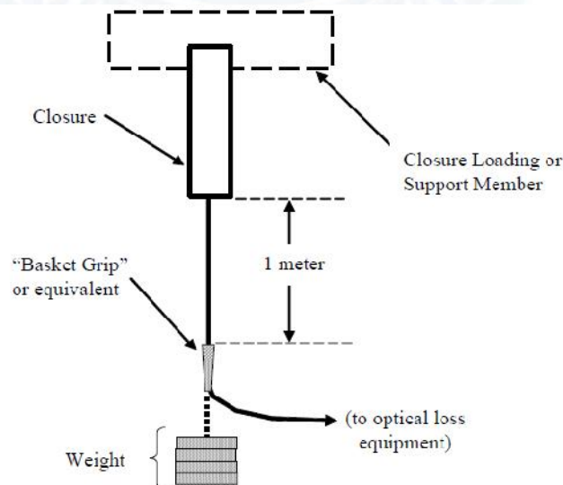
Fig. 1 Fuente: Telcordia GR-771-CORE, ed. 2, punto 5.3.2: Sheath Retention
