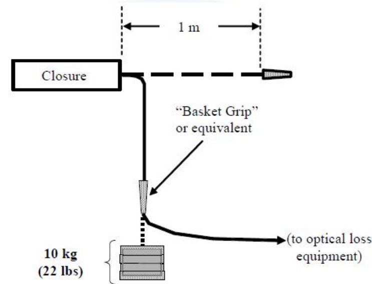
Fig. 2 Fuente: Telcordia GR-771-CORE, ed. 2, punto 5.3.3: Cable Flexing
