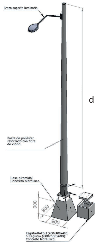
Montaje sobre base piramidal e inserto metálico
