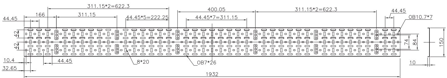
OPGASBC42 Soporte para barra de contactos 42 UR
