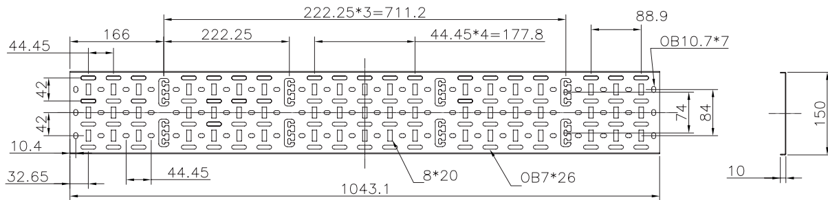
OPGASBC22 Soporte para barra de contactos 22 UR
